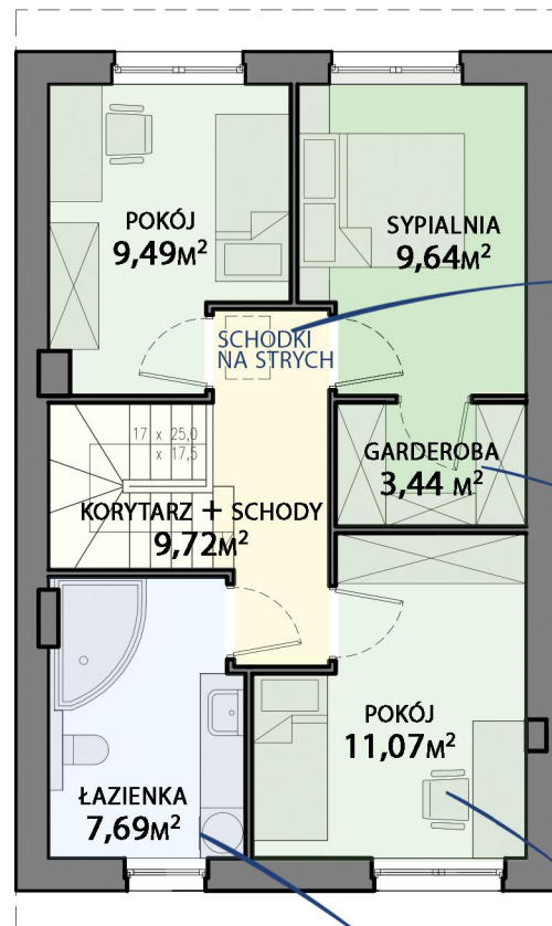
RZUT PIĘTRA
