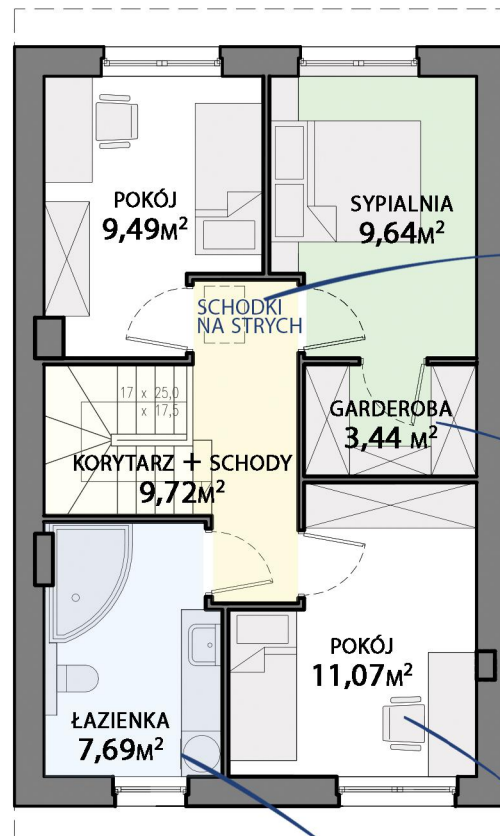
RZUT PIĘTRA
