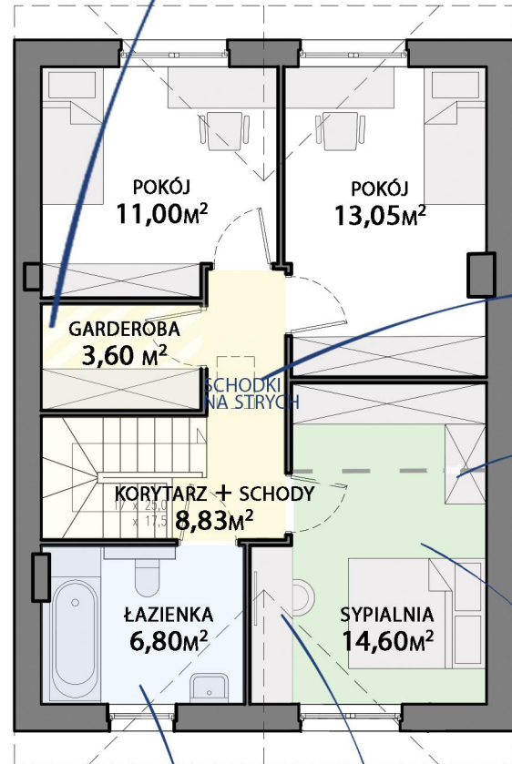
RZUT PIĘTRA
